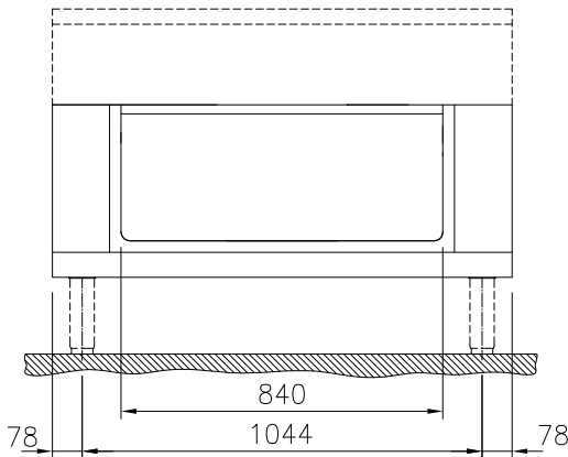
Zij aanzicht
